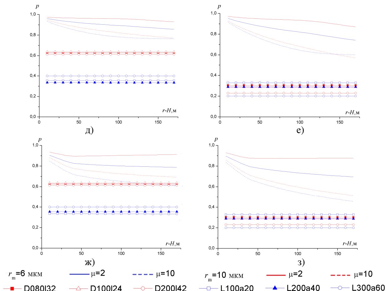
Рисунок 10 – Зависимость степени поляризации лидарного сигнала в приближении двукратного рассеяния от глубины зондирования
