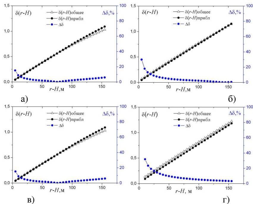
Рисунок 7 – Уровень двукратного рассеяния в лидарном сигнале от однородного облака нижнего яруса ( \mu=2 , r_{\text{mod}}=6 мкм) нижнего яруса: а) H=1 км, \theta_0=3 мрад; б) H=1 км, \theta_0=5 мрад; в) H=2 км, \theta_0=3 мрад; г) H=2 км, \theta_0=5 мрад.
