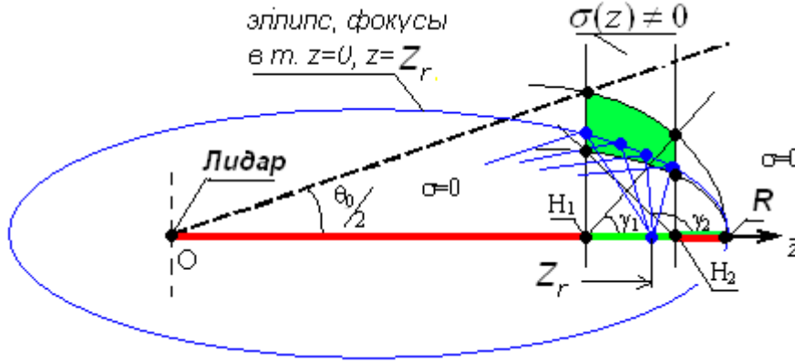
Рисунок 8 – Схема формирования потока двукратного рассеяния облачным слоем
