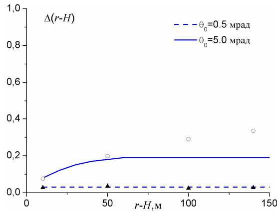
Рисунок 9 – Степень деполаризации лидарного сигнала от облака С1.
