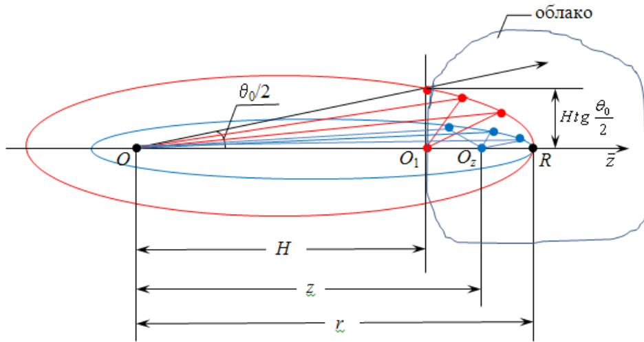
Рисунок 5 – Схема формирования потока двукратно рассеянного назад излучения от облака, когда глубина зондирования не превышает радиуса поперечного сечения диаграммы направленности приёмной системы лидара на входе в облако ( r-H \leq H \tan(\theta_0/2) )
