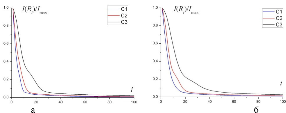
Рисунок 4 – Распределение нормированной интенсивности двукратного рассеяния в плоскости регистрации для моделей облаков С1, С2, С3 при длине волны: а) 450 нм; б) 700 нм
