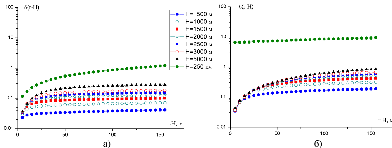
Рисунок 2 – Зависимость \delta(r-H) для различной дальности облака H при двух значениях угла поля зрения приемной системы лидара: а) \theta_0=0.1 мрад, б) \theta_0=0.5 мрад.
