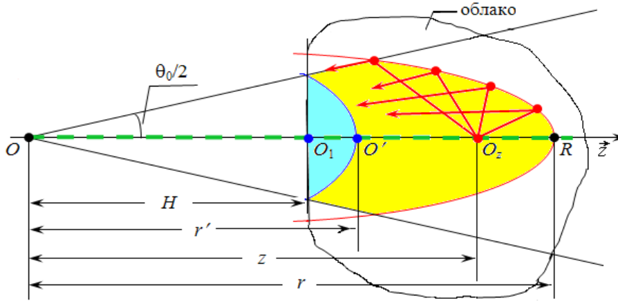
Рисунок 6 – Схема формирования потока двукратного рассеяния при r - H \geq Htg\frac{\theta_0}{2}
